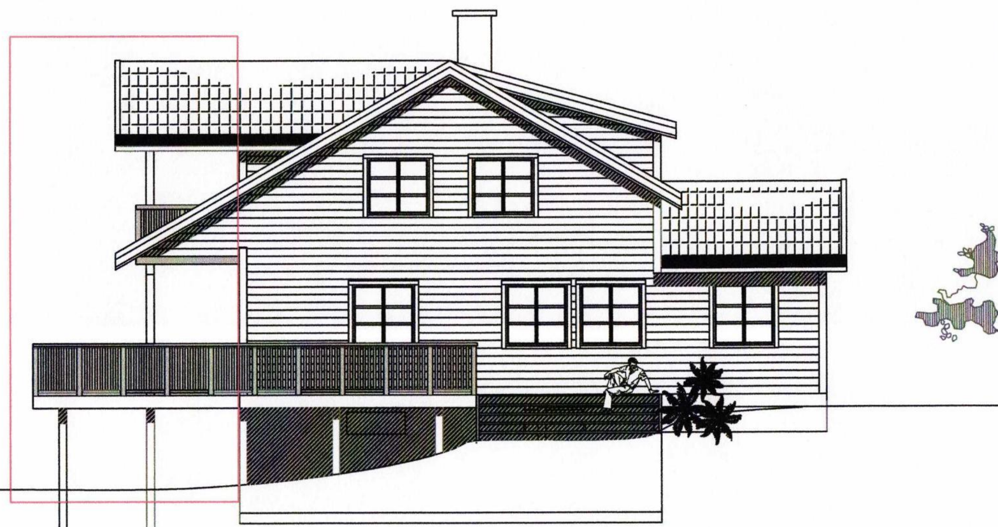
Fasade: Øst
