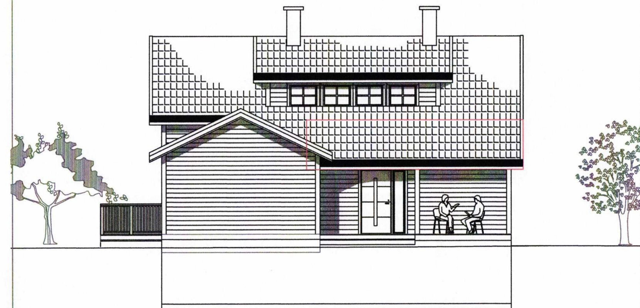
Fasade: Nord
